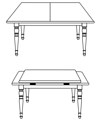
Art. 912/A Tavolo a libro Extensible table L. 100 P. 100 H. 78 (aperto cm 100x200)
